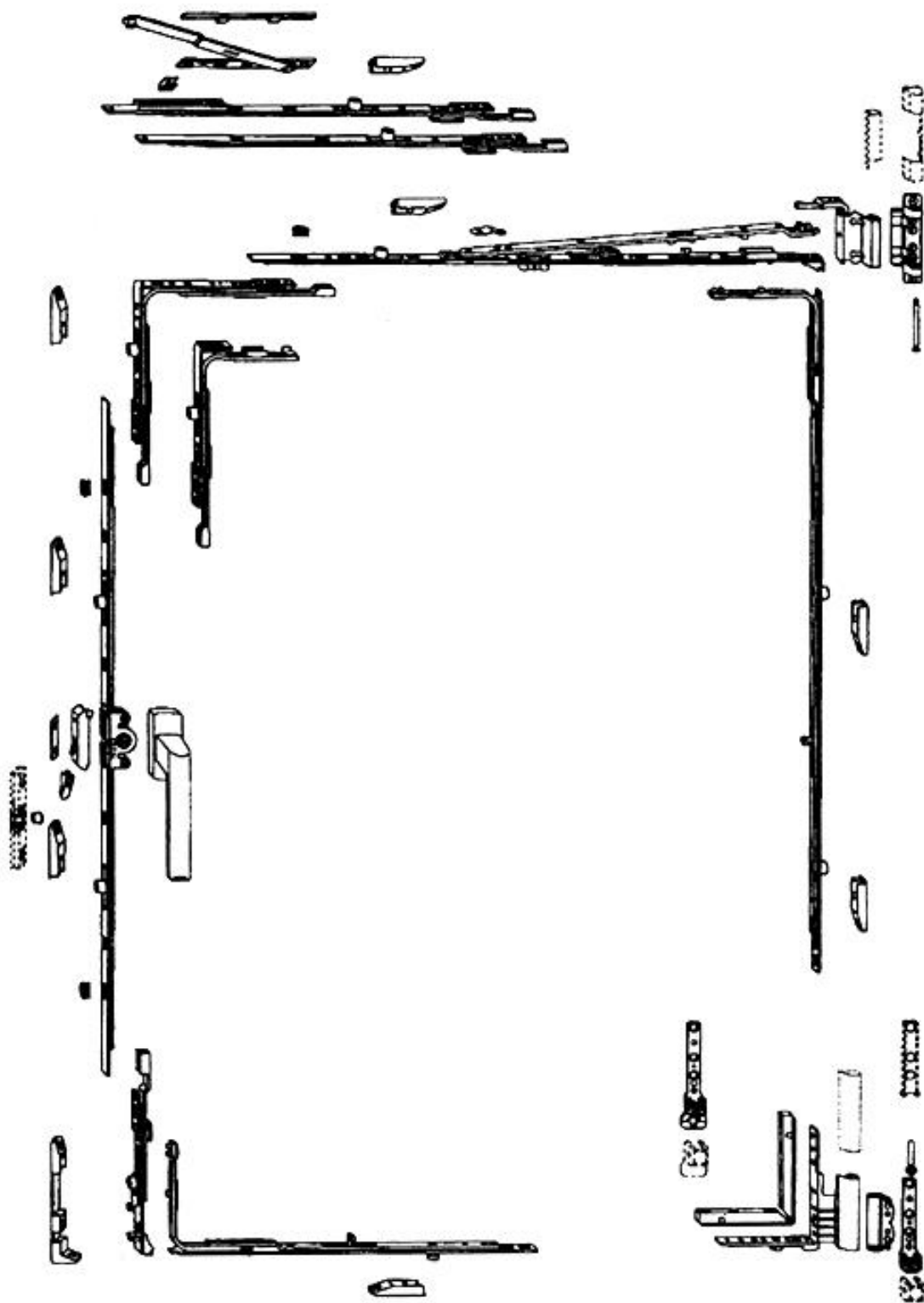
Рисунок Б.3 - Устройство поворотно-откидное
