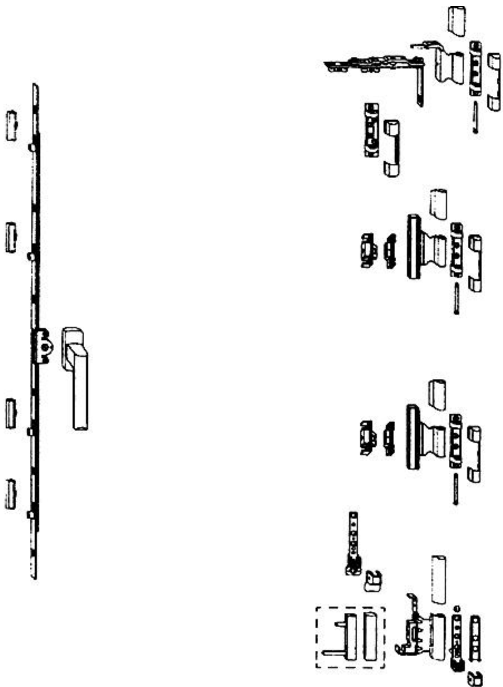
Рисунок Б.1 - Устройство поворотное
